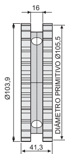
SECCIÓN A-A
