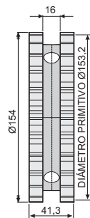
SECCIÓN A-A
