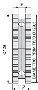
SECCIÓN A-A
