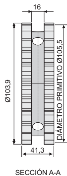
SECCIÓN A-A
