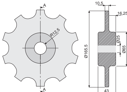
SECCIÓN A-A
