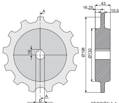
SECCIÓN A-A
