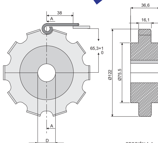
SECCIÓN A-A
