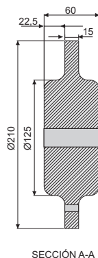
SECCIÓN A-A
