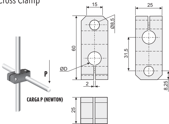
Mordaza En Cruz Cross Clamp
