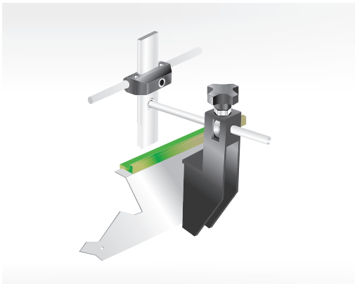
Mordaza Ajustable Perfil Cuadrado Adjustable Clamp
